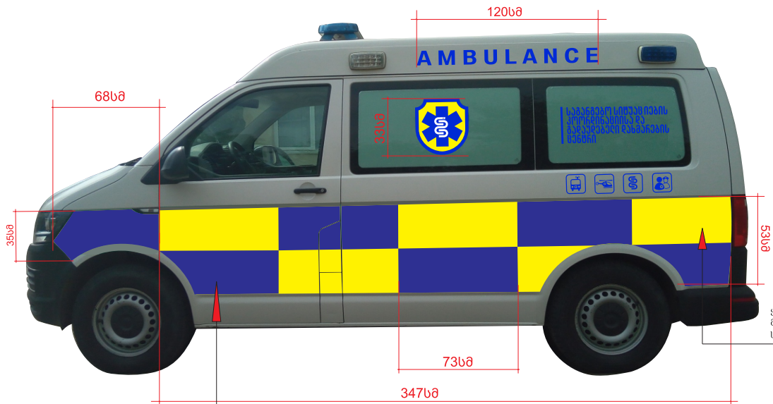
ლურჯი თვითწებავი ვინილი ეკრობა ვეითელი ვინილის ზემოიდან. გაკვრა იწყება წინა მხრიდან და ყველა ლურჯი კუბიკი (ბოლოს გარდა) არის 73 სმ. ბოლო კუბიკი იჭრება უკანა სანაითის კონტურზე. ლურჯი და ყვითელი არეები უნდა იყოს თანაბარი სიძლიის
