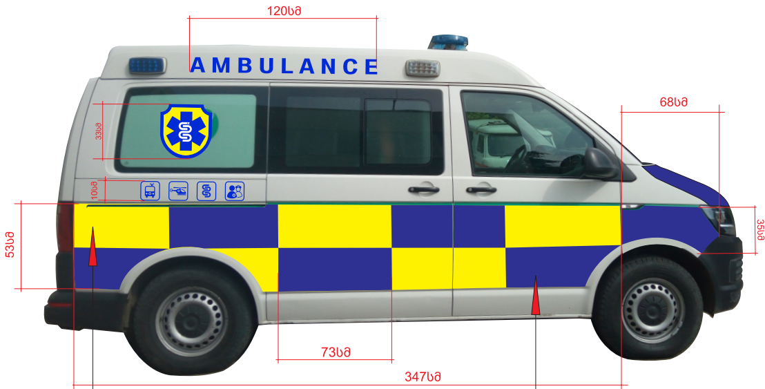
ლურჯი თვითწებავი ვინილი ეკრობა ვეითელი ვინილის ზემოიდან. გაკვრა იწყება წინა მხრიდან და ყველა ლურჯი კუბიკი (ბოლოს გარდა) არის 73 სმ. ბოლო კუბიკი იჭრება უკანა სანაითის კონტურზე. ლურჯი და ყვითელი არეები უნდა იყოს თანაბარი სიძლიის
